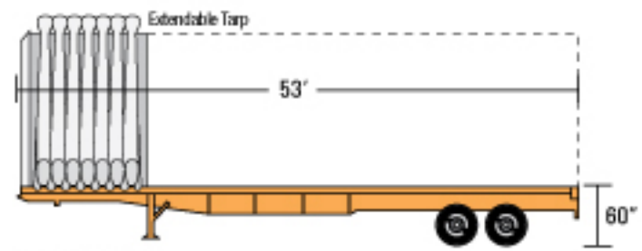
Conestoga
